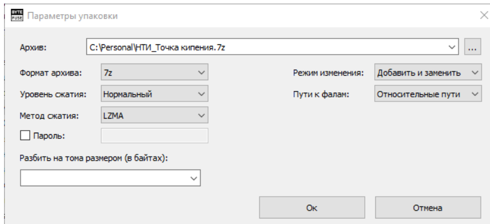
Рисунок 4. Окно Параметры упаковки
