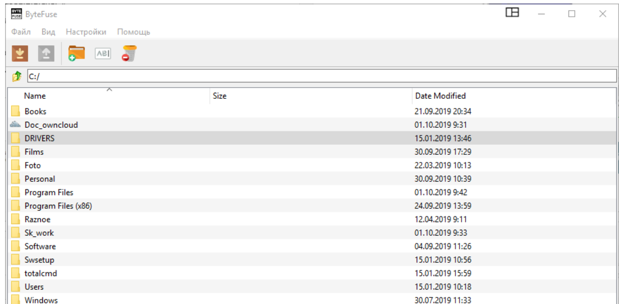
Рисунок 1. Главное окно
