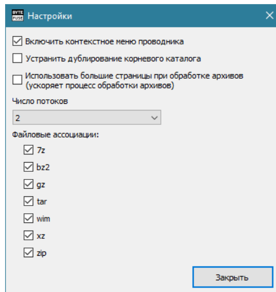
Рисунок 2. Меню настройки
